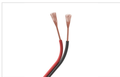
Артикул 026348 Шлейф для питания и управления одноцветными светодиодными лентами. 2 проводника, калибр проводника 18AWG, сечение проводника 0.
