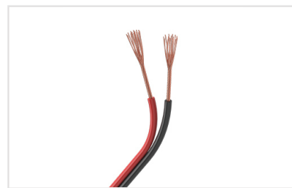
Артикул 033152 Шлейф для питания и управления одноцветными светодиодными лентами. 2 проводника, калибр проводника 16AWG, сечение проводника 1.
