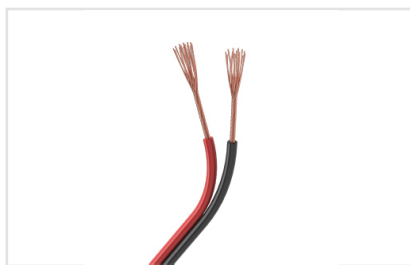
Артикул 026349 Шлейф для питания и управления одноцветными светодиодными лентами. 2 проводника, калибр проводника 20AWG, сечение проводника 0.
